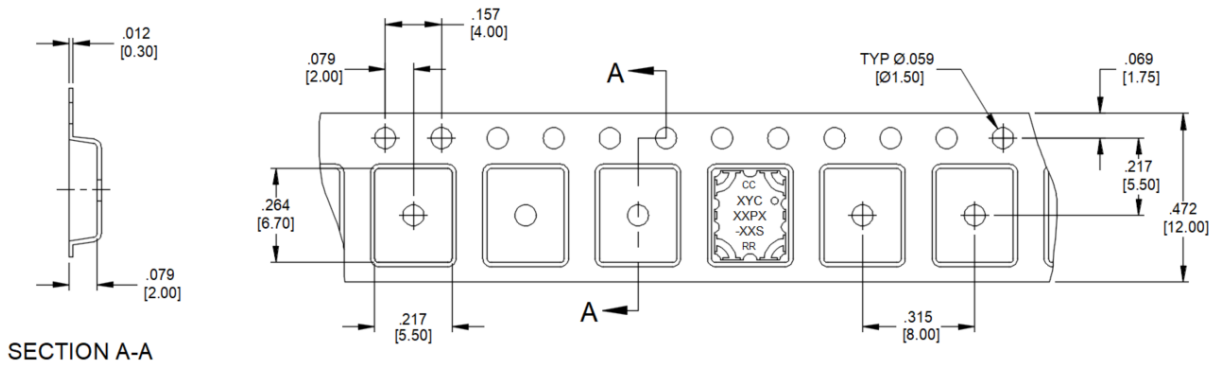
SECTION A-A
