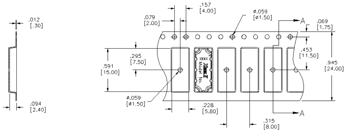
SECTION A-A
