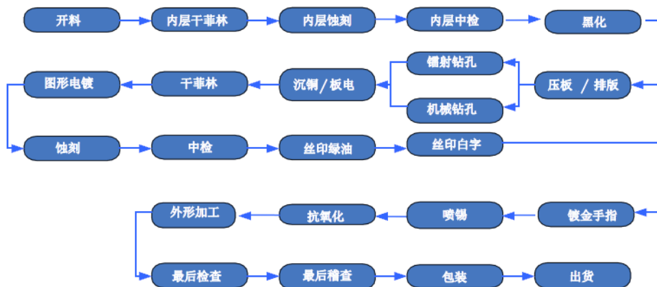
图 3.4-3 PCB 线路板生产工艺（1994 年-2007 年）
