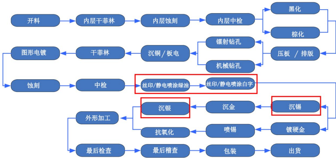
图 3.4-4 PCB 线路板生产工艺（2007 年至今）
