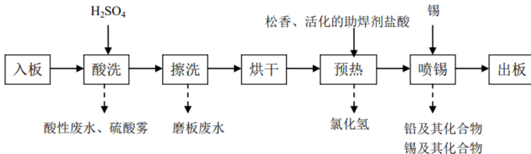
图 3.4-19 喷锡工艺流程及产排污节点图
