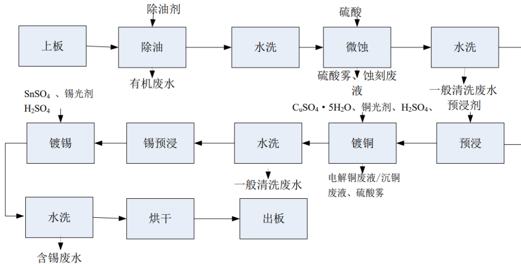
图 3.4-15 脉冲图形电镀工艺流程及产排污节点图
