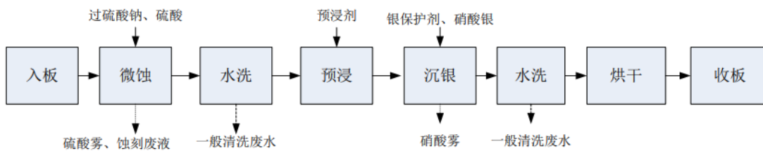
图 3.4-23 沉银工艺流程及产排污节点图
