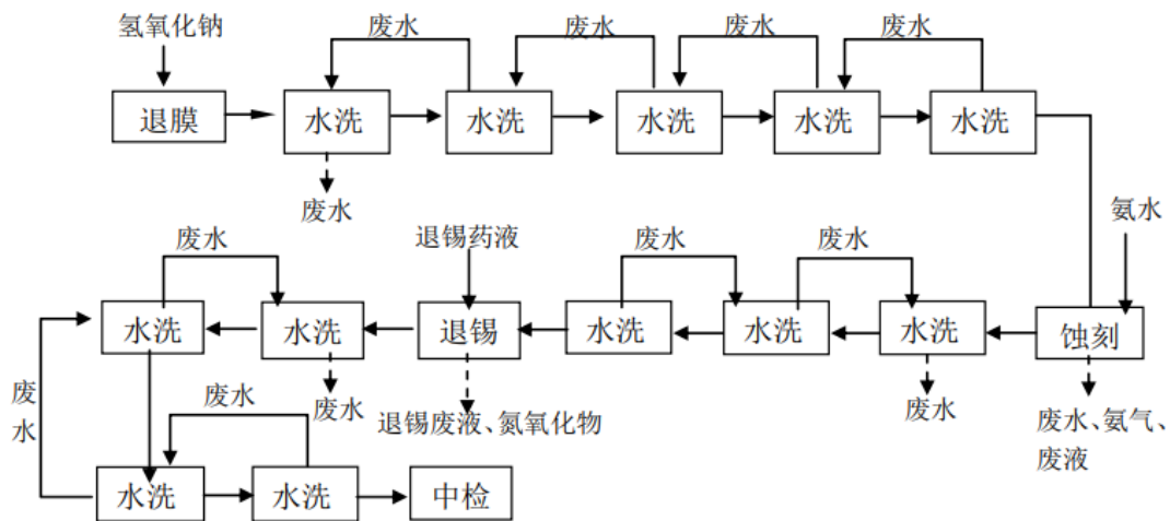
图 3.4-16 项目蚀刻工艺流程及产排污节点图
