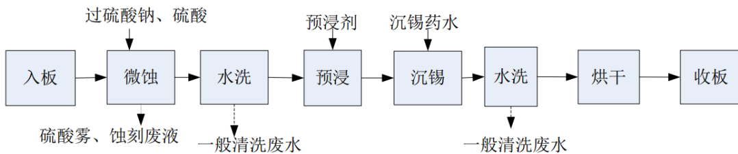
图 3.4-21 沉锡工艺流程及产排污节点图
