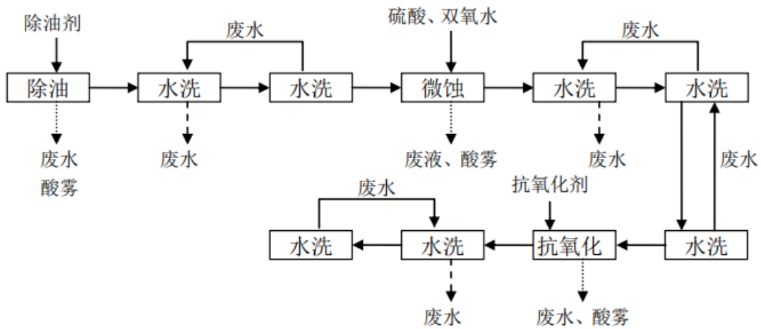
图 3.4-20 镀硬金工艺流程及产排污节点图
