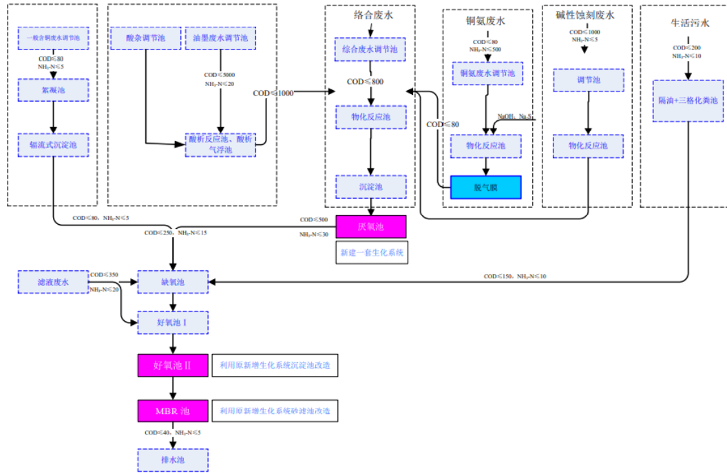
图 3.5-3 污水处理流程图 (COD、氨氮)
