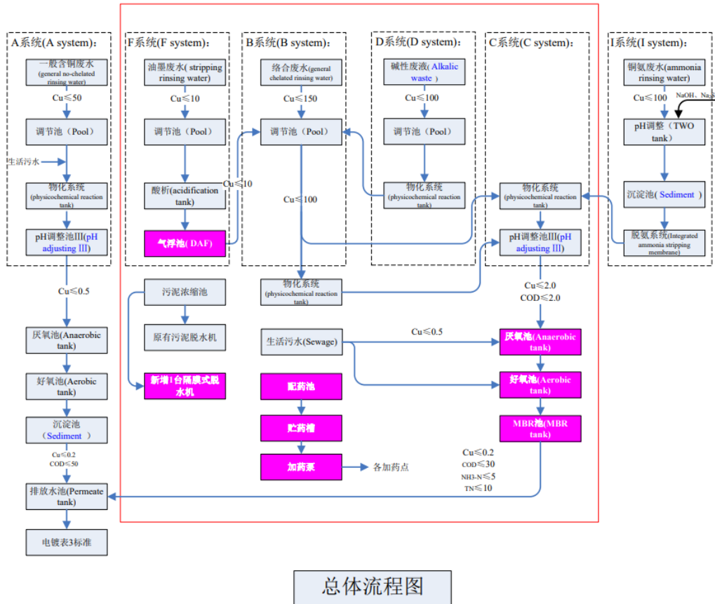
图 3.5-4 污水处理流程图 (Cu 2+ )
